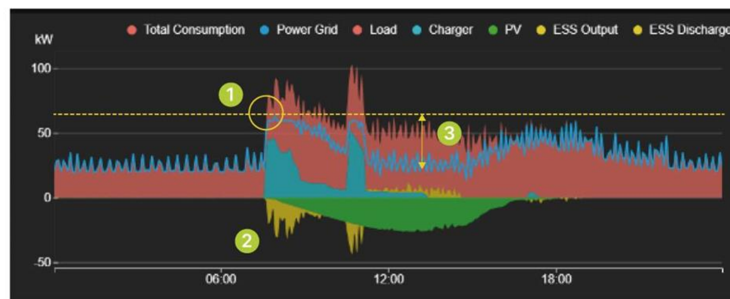
導入後 每日負載曲線
