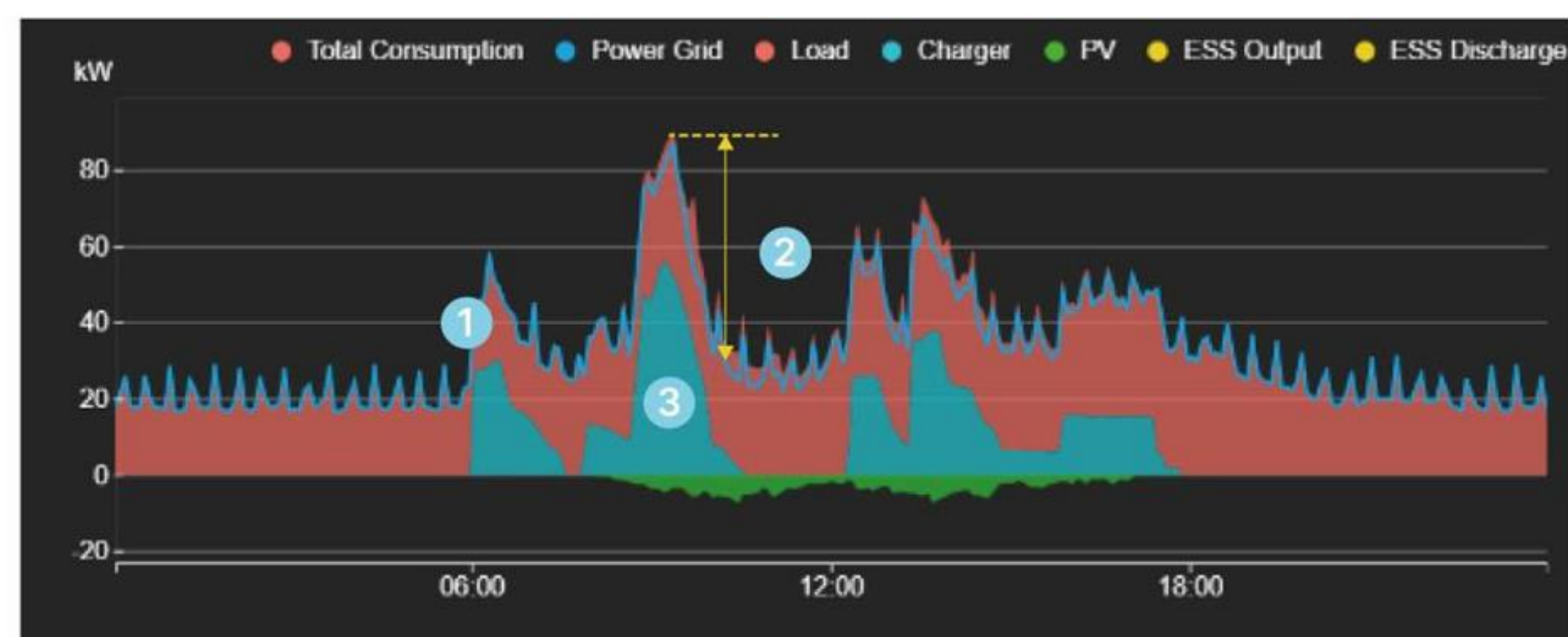
導入前 每日負載曲線
